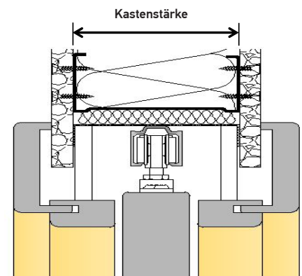
Darstellung: Schiebetürkasten für Gips mit Umfassungszarge ML = DGL + 97 mm
