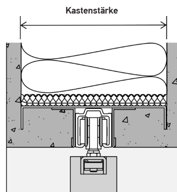
Darstellung: Schiebetürkasten verputzt mit Schiene (geringe Einbauhöhe) ML = DGL + 47 mm bis 80 kg ML = DGL + 54 mm bis 140 kg
